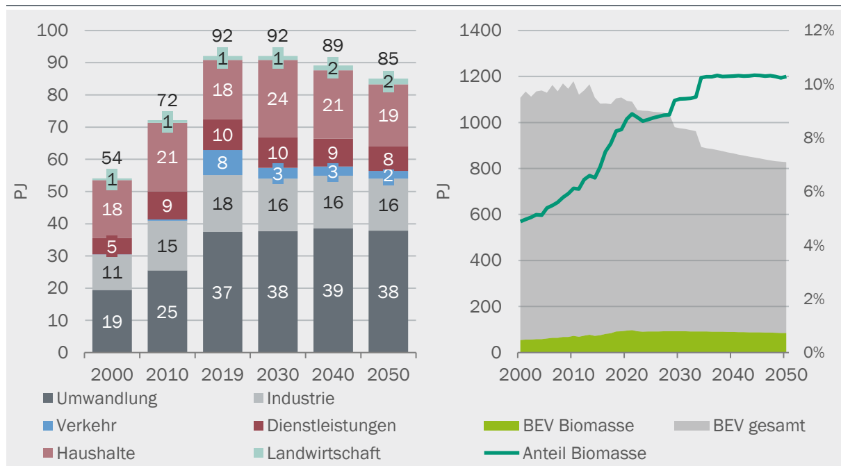
Abbildung 15: Biomasseeinsatz im Szenario Weiter wie bisher
